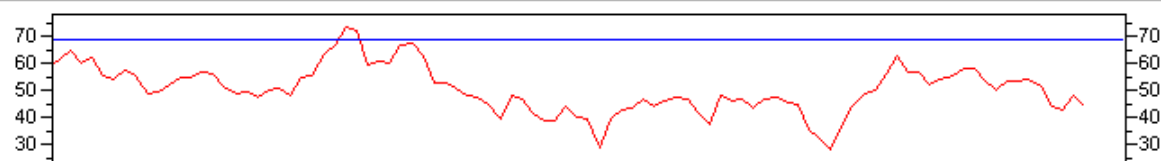
— ИнтерРАОao [RSI]
