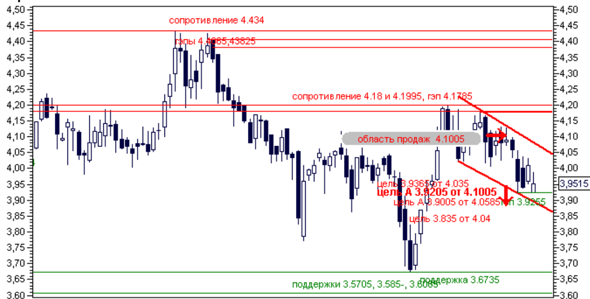
— ИнтерРАОao [Price]
